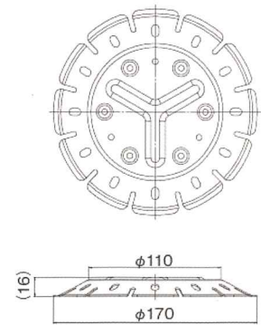
押さえ金具
